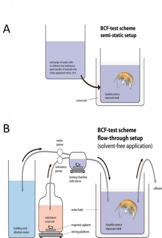
Abb. 2. HYBIT Ringtestprotokoll: Schematischer Überblick über den Versuchsaufbau des semi-statischen Tests (A) und des Durchflusstests (B).
